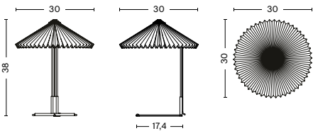
Matin Table Lamp 300
