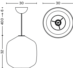
Buoy Glass Pendant 300
