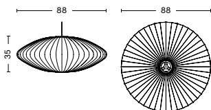
Nelson Saucer Bubble Pendant L
